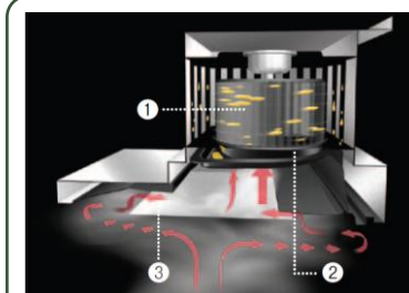
スーパークリーンフード構造図 ①シロッコファン②オイルバック③整流板
